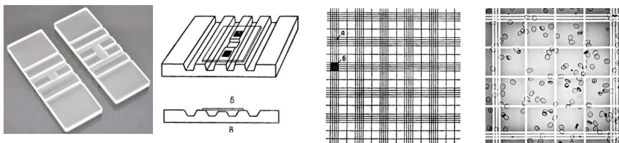
Рис. 1. Камера Горяева-Тома для подсчета количества микроорганизмов
